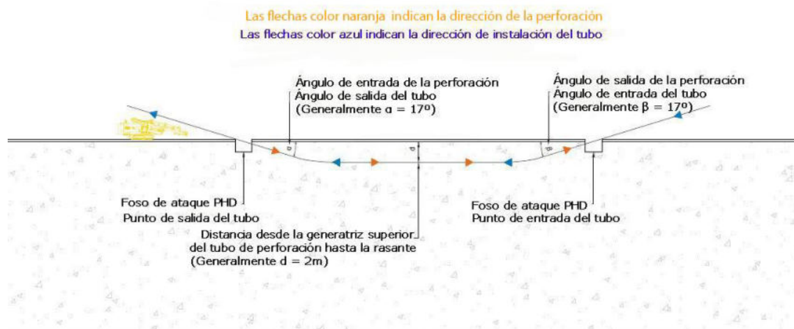
Figura 2. Esquema de perforación e instalación del tubo
